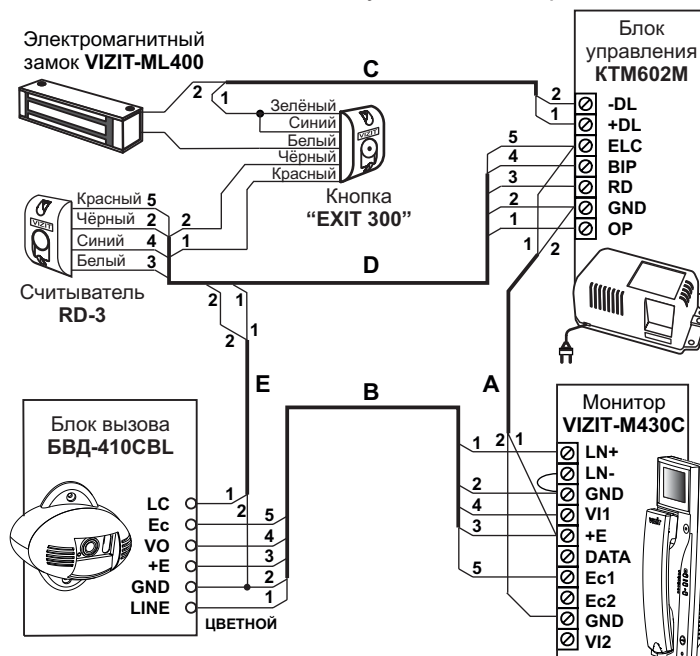
Рисунок 7 - Схема соединений БВД-410CBL с блоком коммутации монитора БКМ-440
